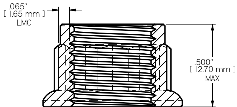
SECTION A-A 3X SCALE
